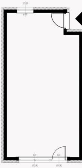
PARTER 45,51 m 2
